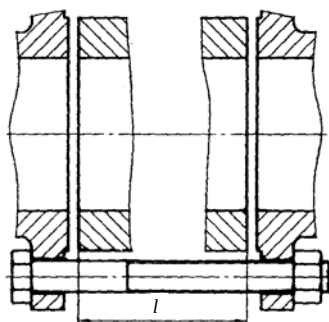
图3 对夹连接阀门结构长度
