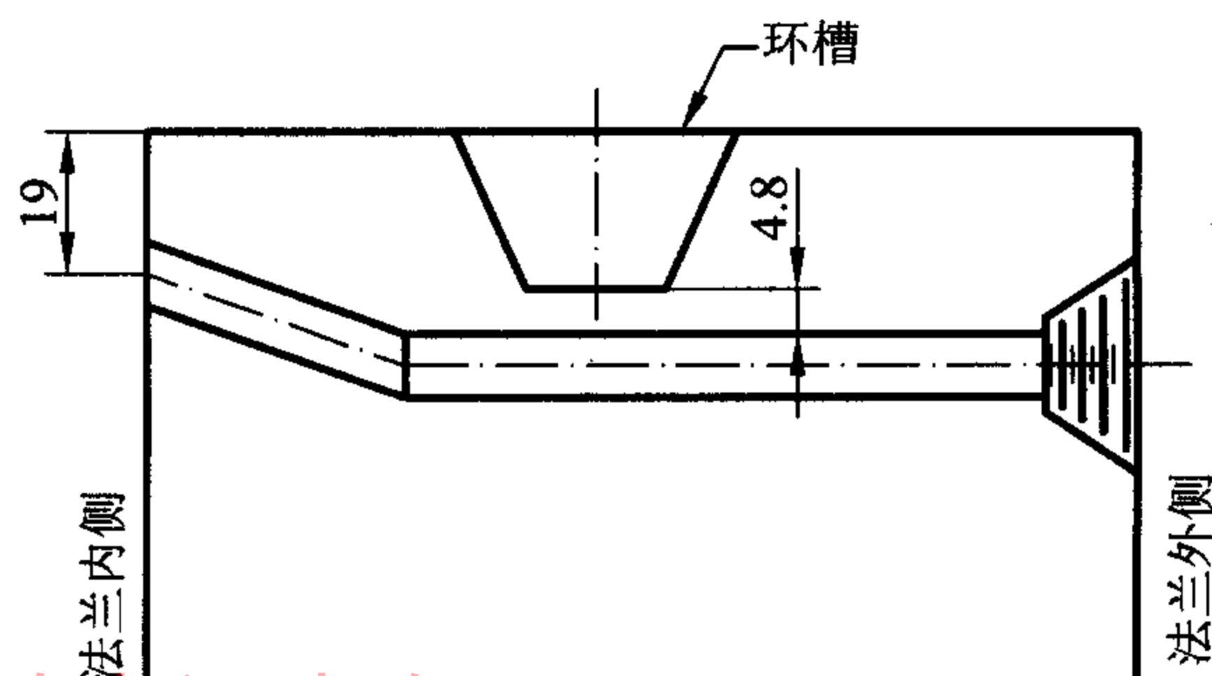
图 A.7.1 带颈对焊孔板法兰结构示意图(径向测压孔)
