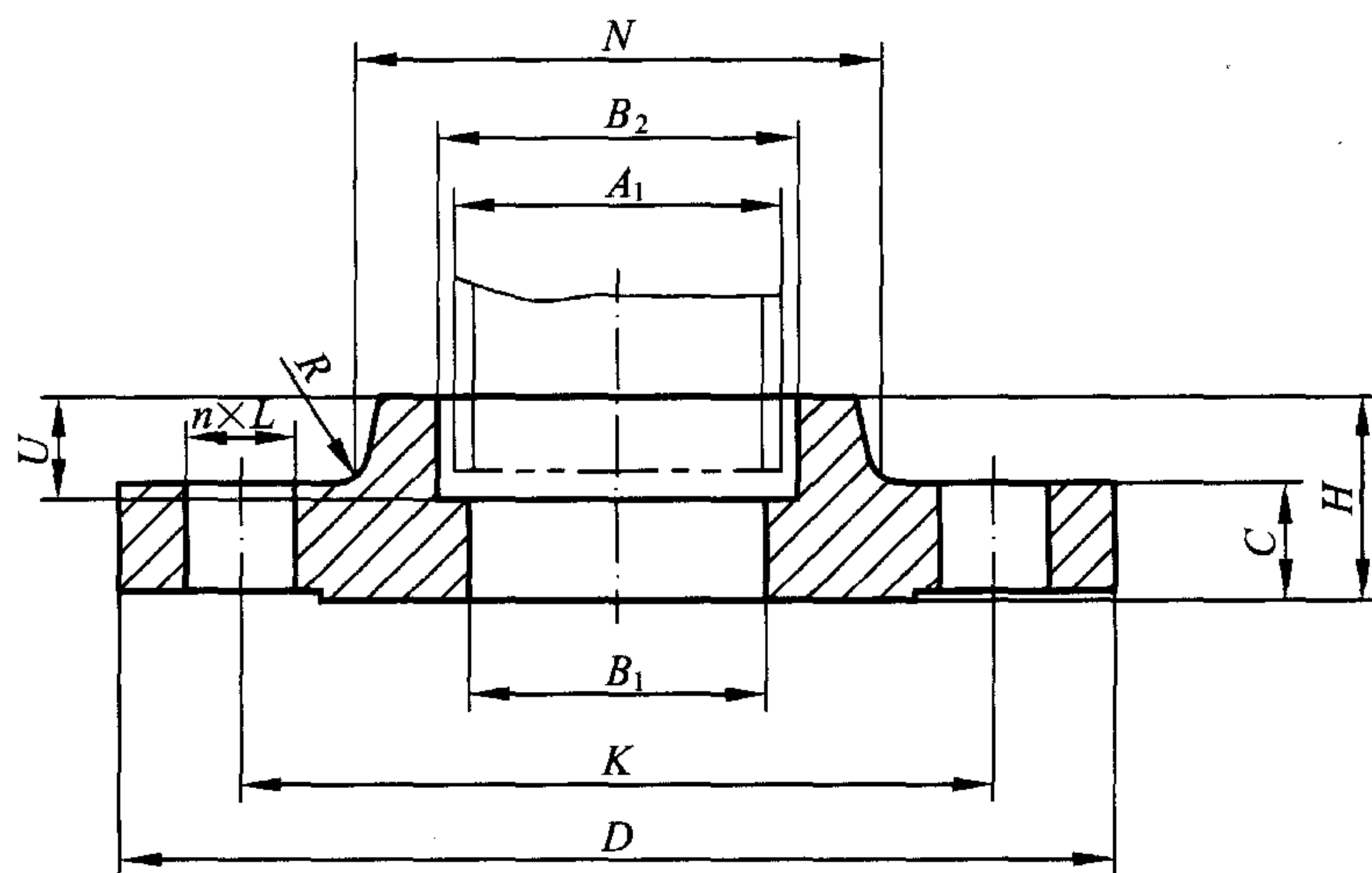
图 8.2.5 承插焊钢制管法兰
