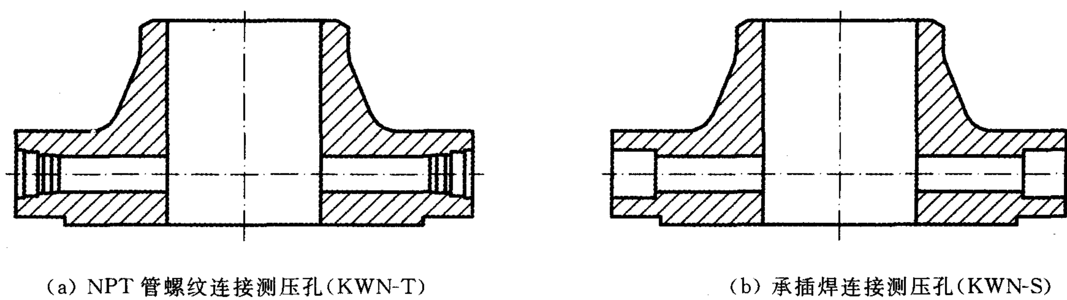
图 A.3-1 带颈对焊孔板法兰类型
