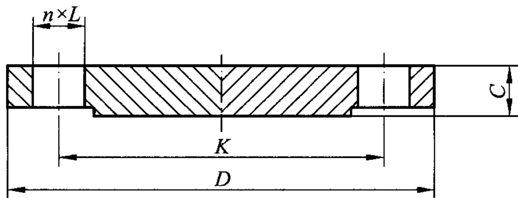
图 8.2.9 钢制管法兰盖
