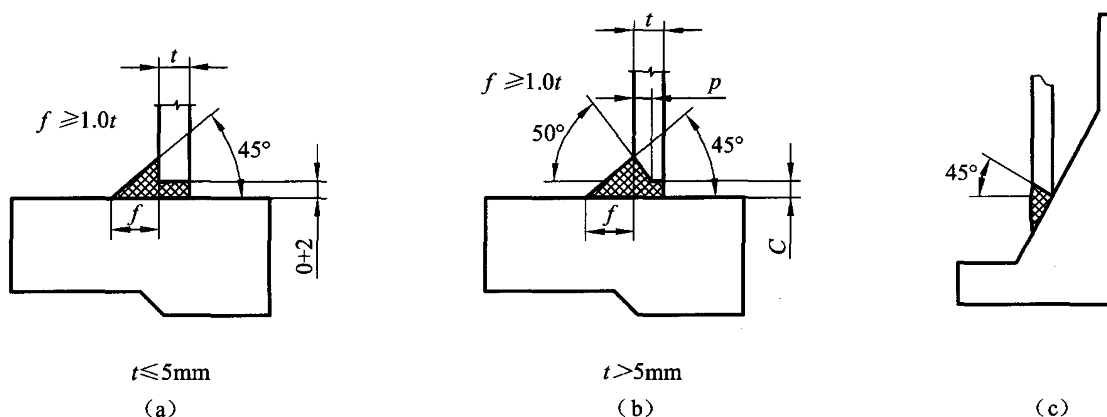
图 B.7.2 外管与夹套法兰的焊缝尺寸
