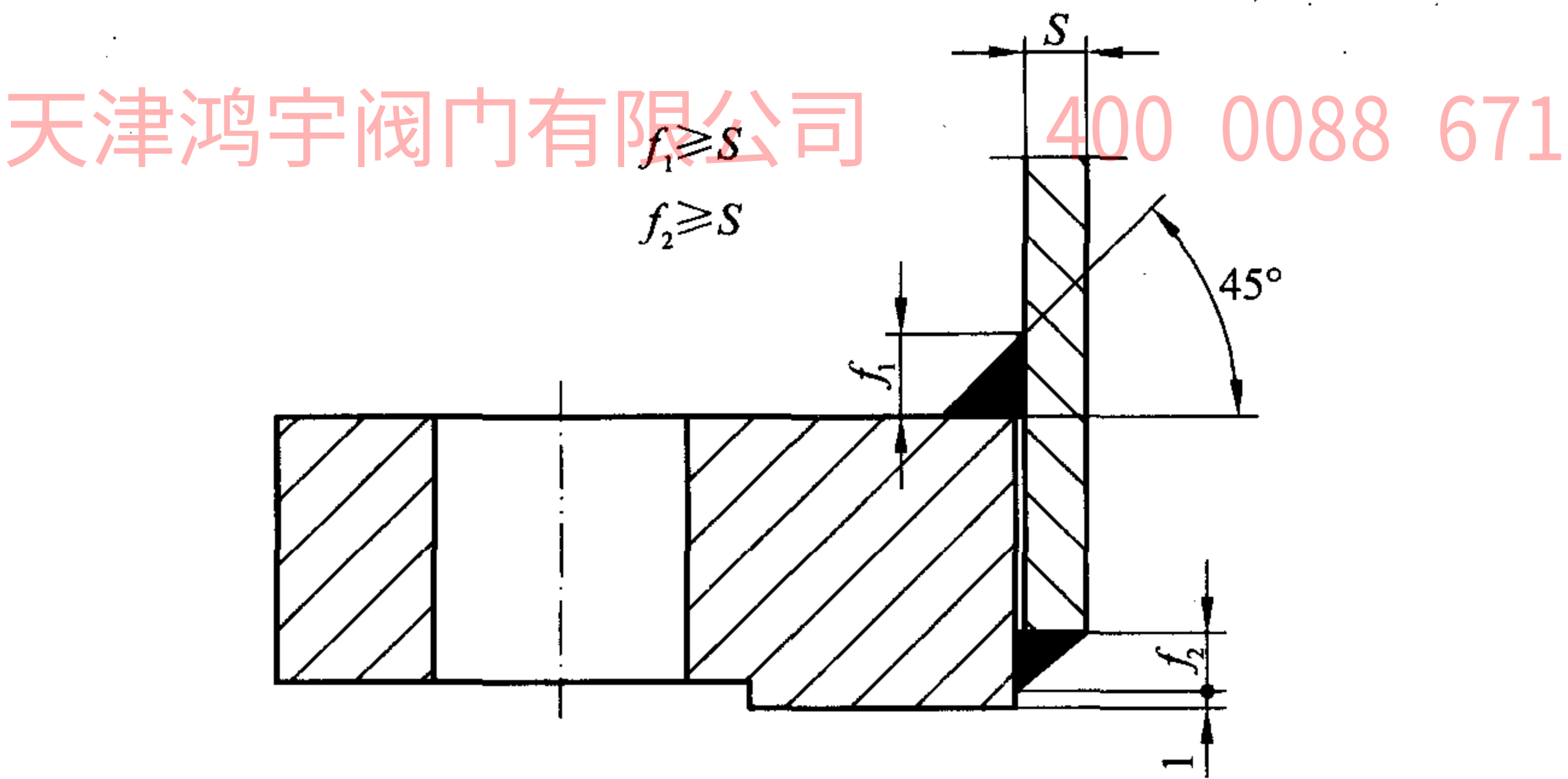
图 9.1.1 板式平焊法兰或平焊环与钢管连接的焊接接头
