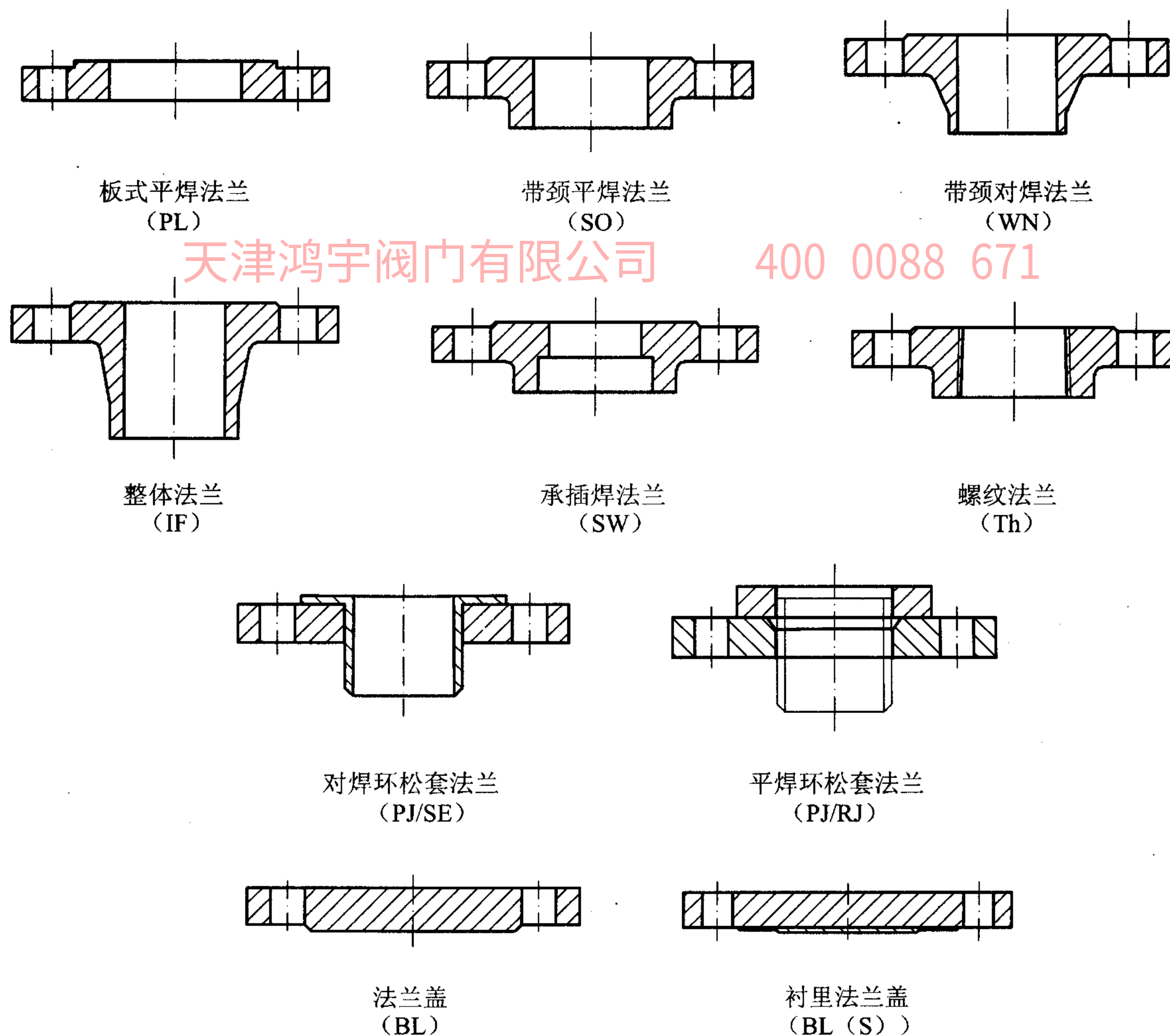
图 3.1.1 法兰类型及其代号
