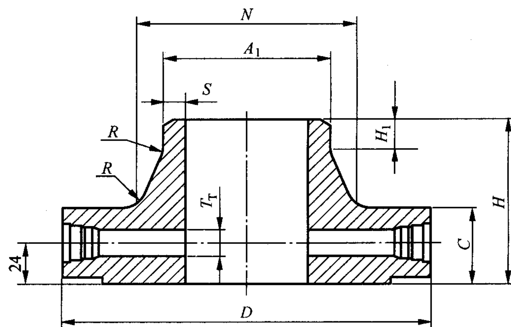
图 A.8.2 带颈对焊孔板法兰
