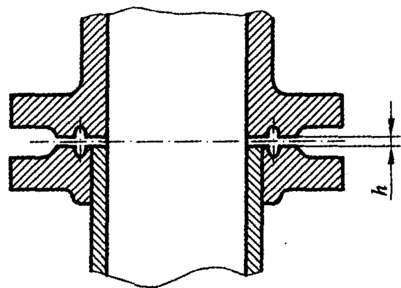
图 E 环连接面法兰
