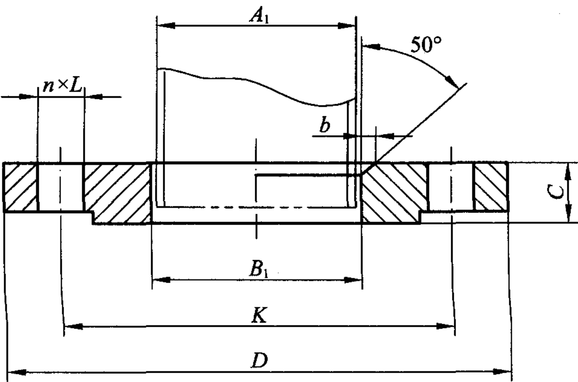
图 8.2.1 板式平焊钢制管法兰
