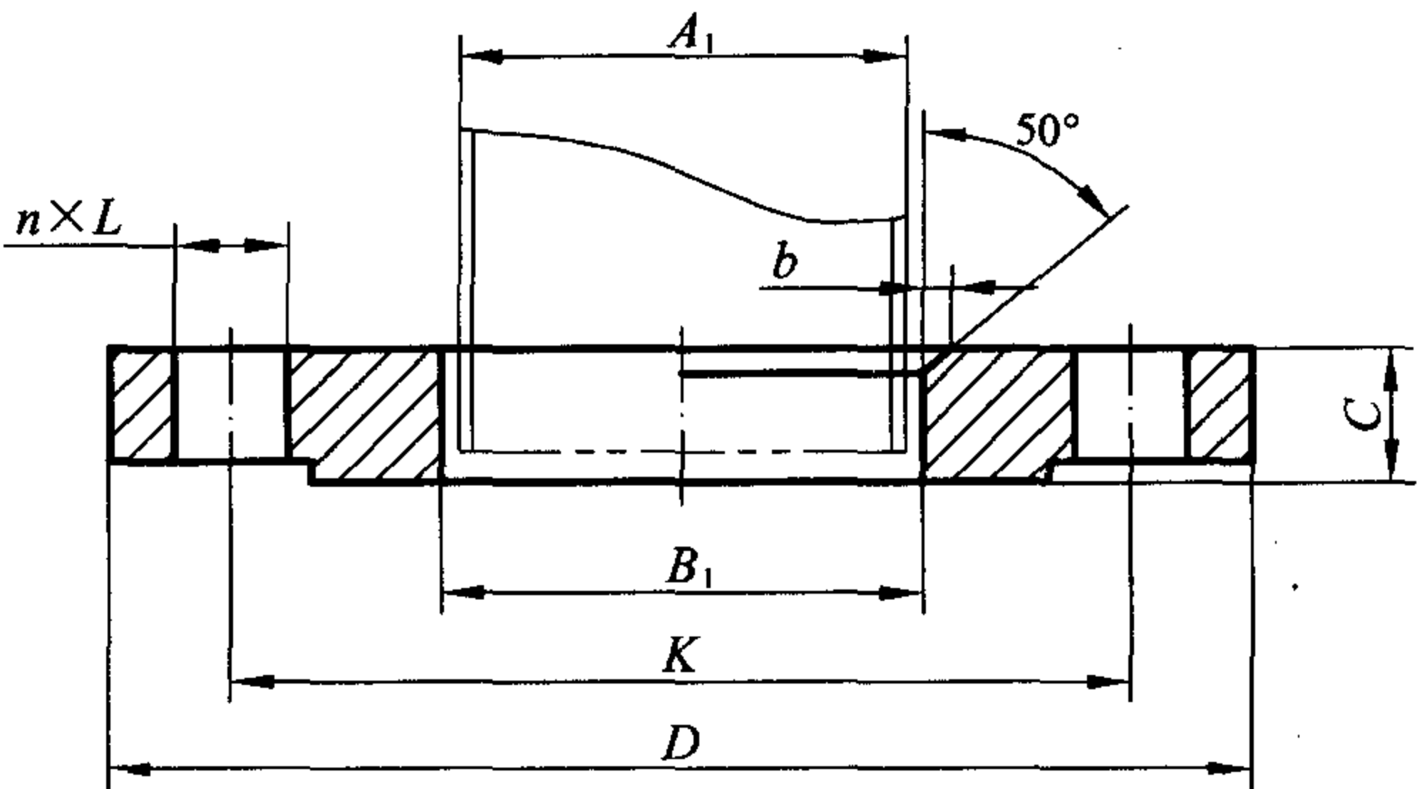
图 B.6.2-1 板式平焊钢制夹套法兰
