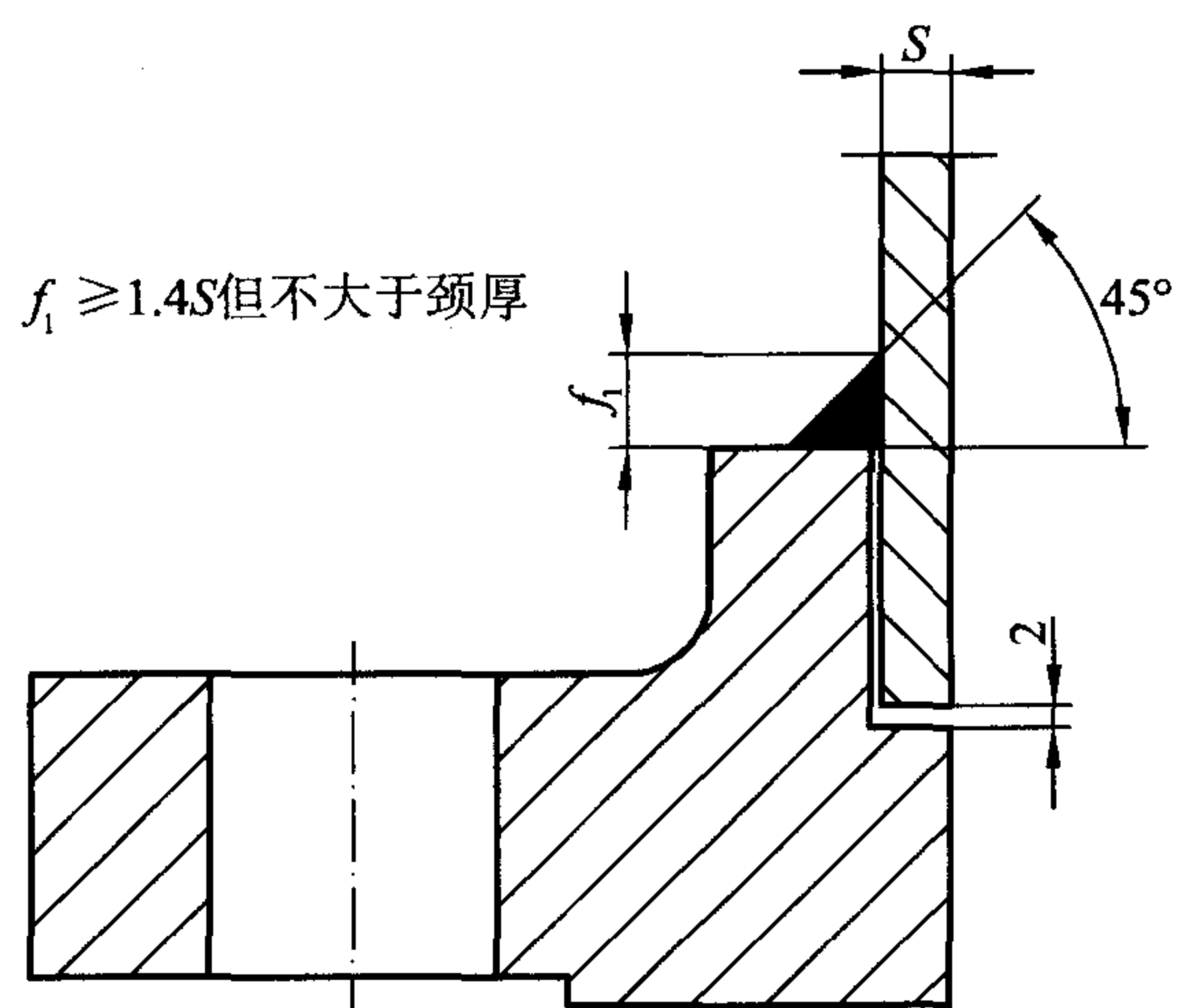
图 9.3 承插焊法兰与钢管连接的焊接接头
