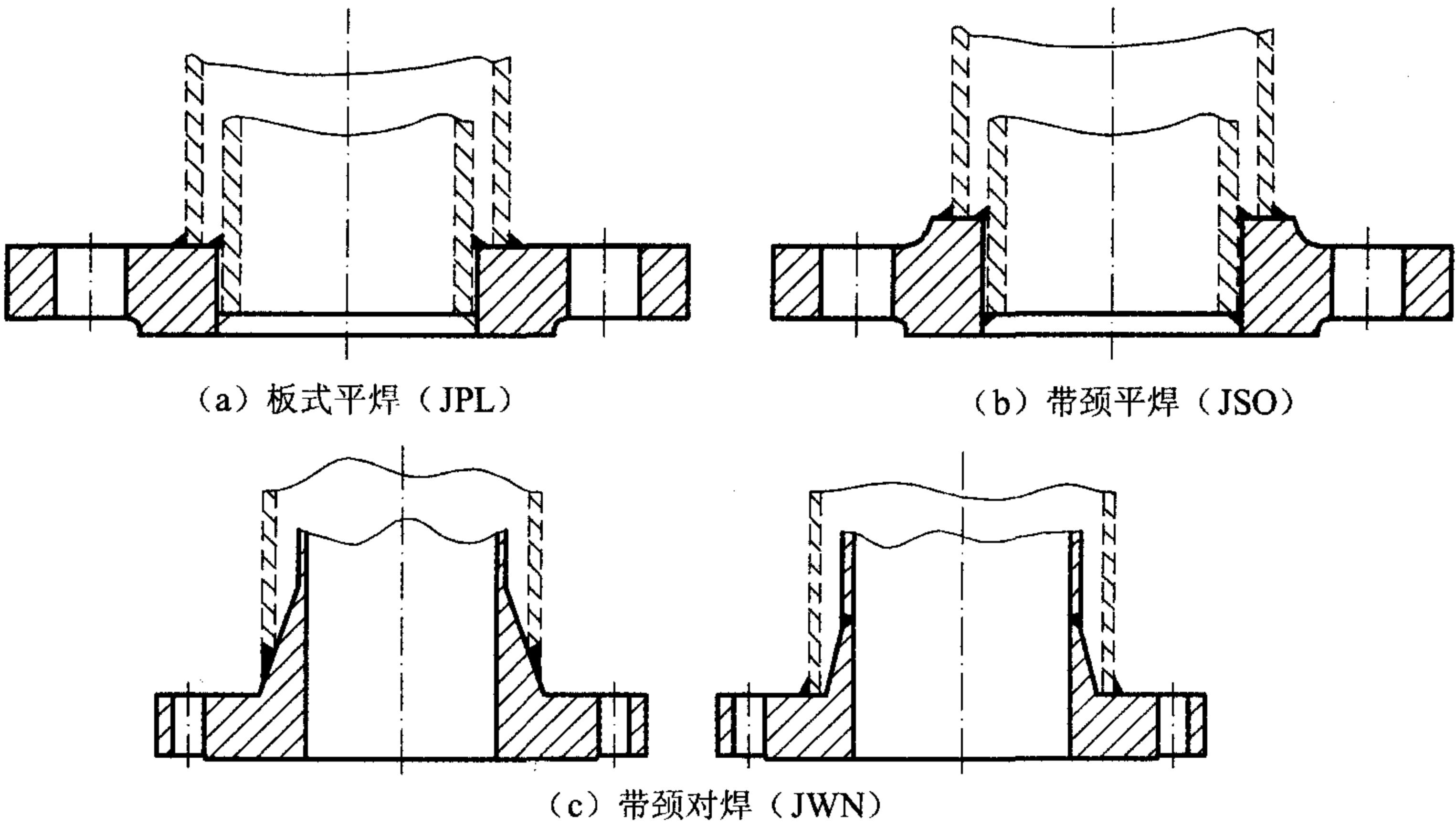
图 B.3.1 夹套法兰类型
