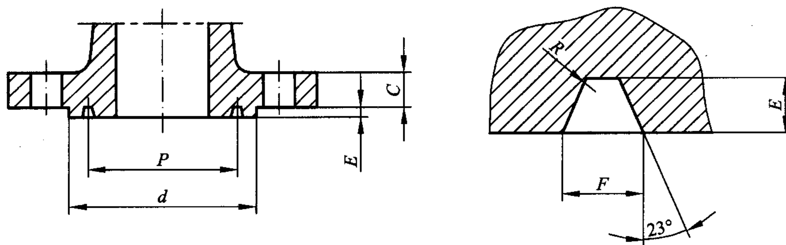
图 3.2.5-2 环连接面的密封面尺寸
