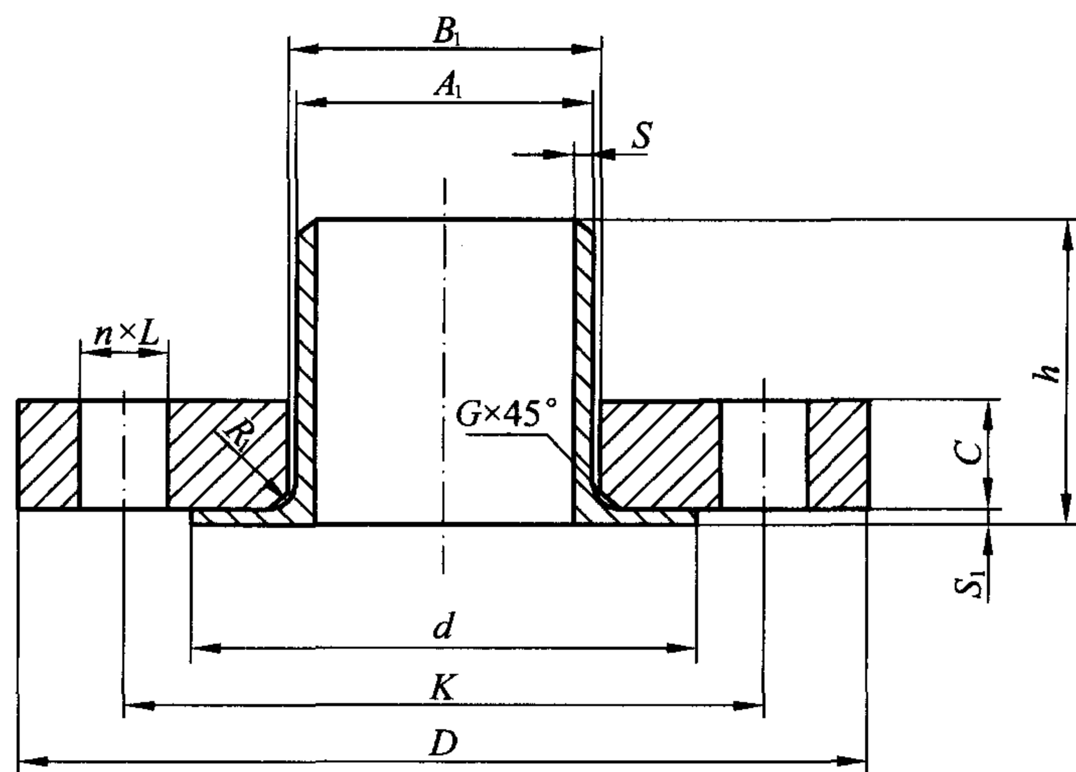
图 8.2.7 对焊环松套钢制管法兰
