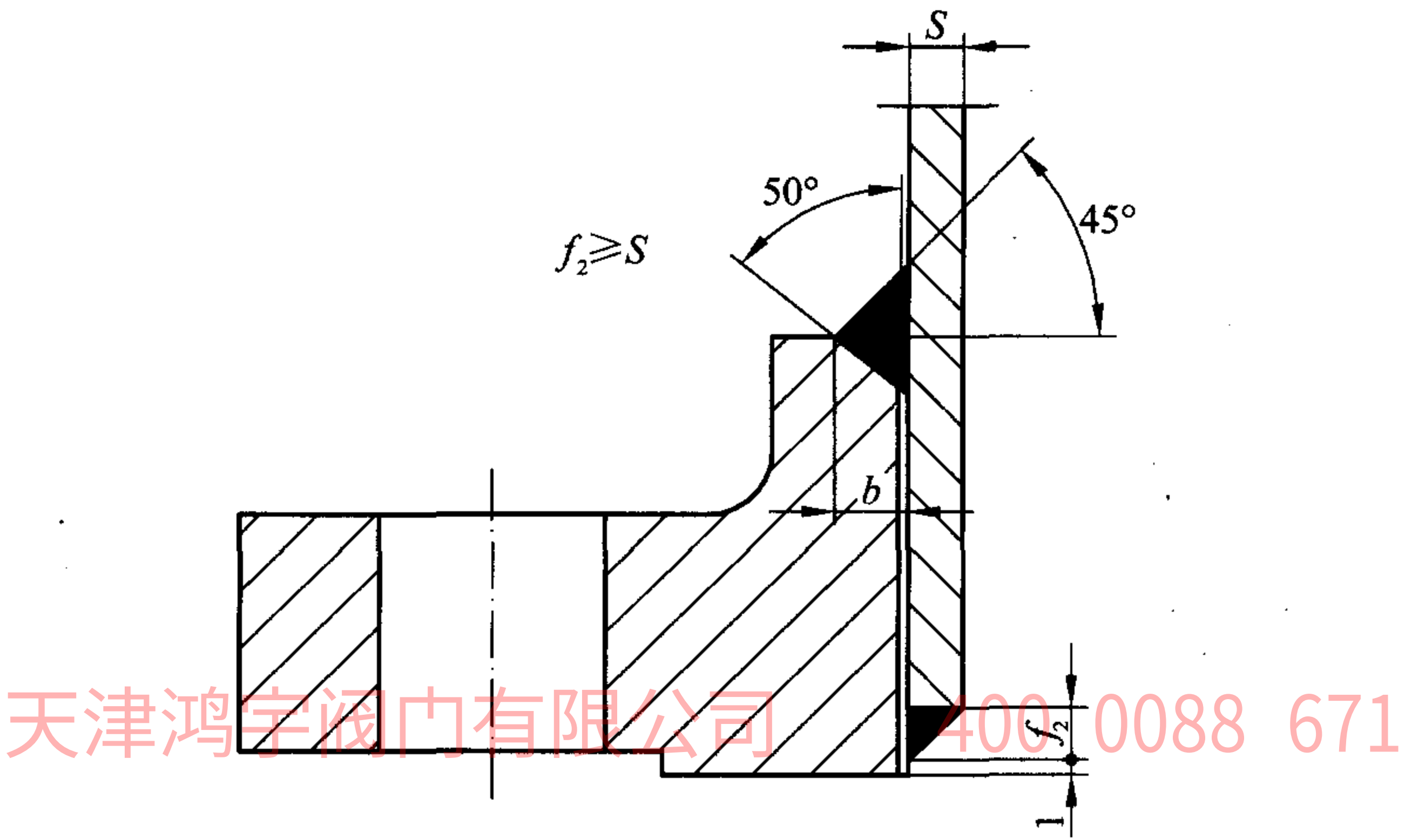
图 9.2.2 带颈平焊法兰与钢管连接的焊接接头
