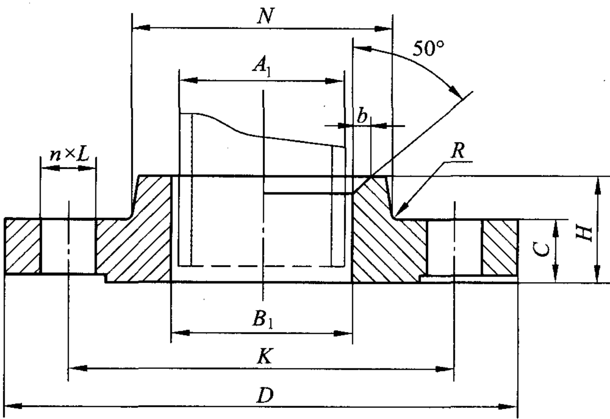
图 B.6.2-2 带颈平焊钢制夹套法兰
