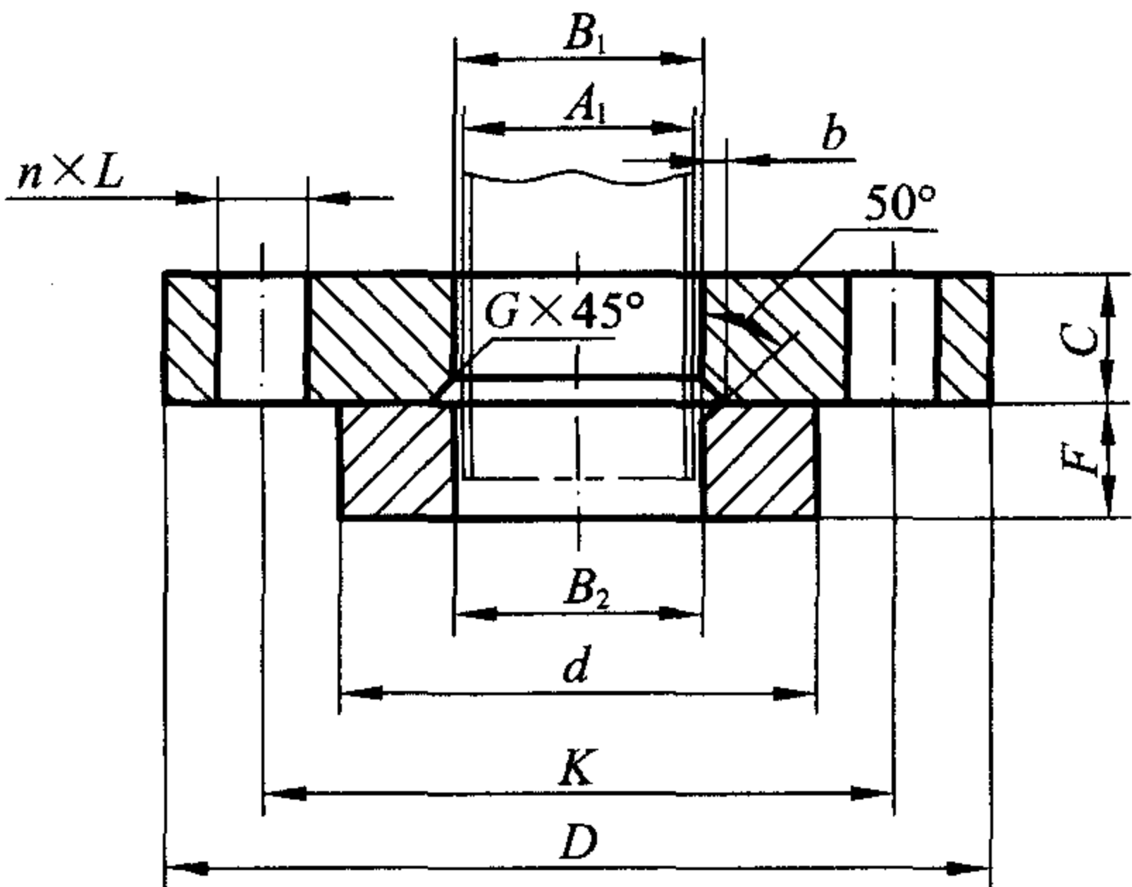
图 8.2.8 平焊环松套钢制管法兰
