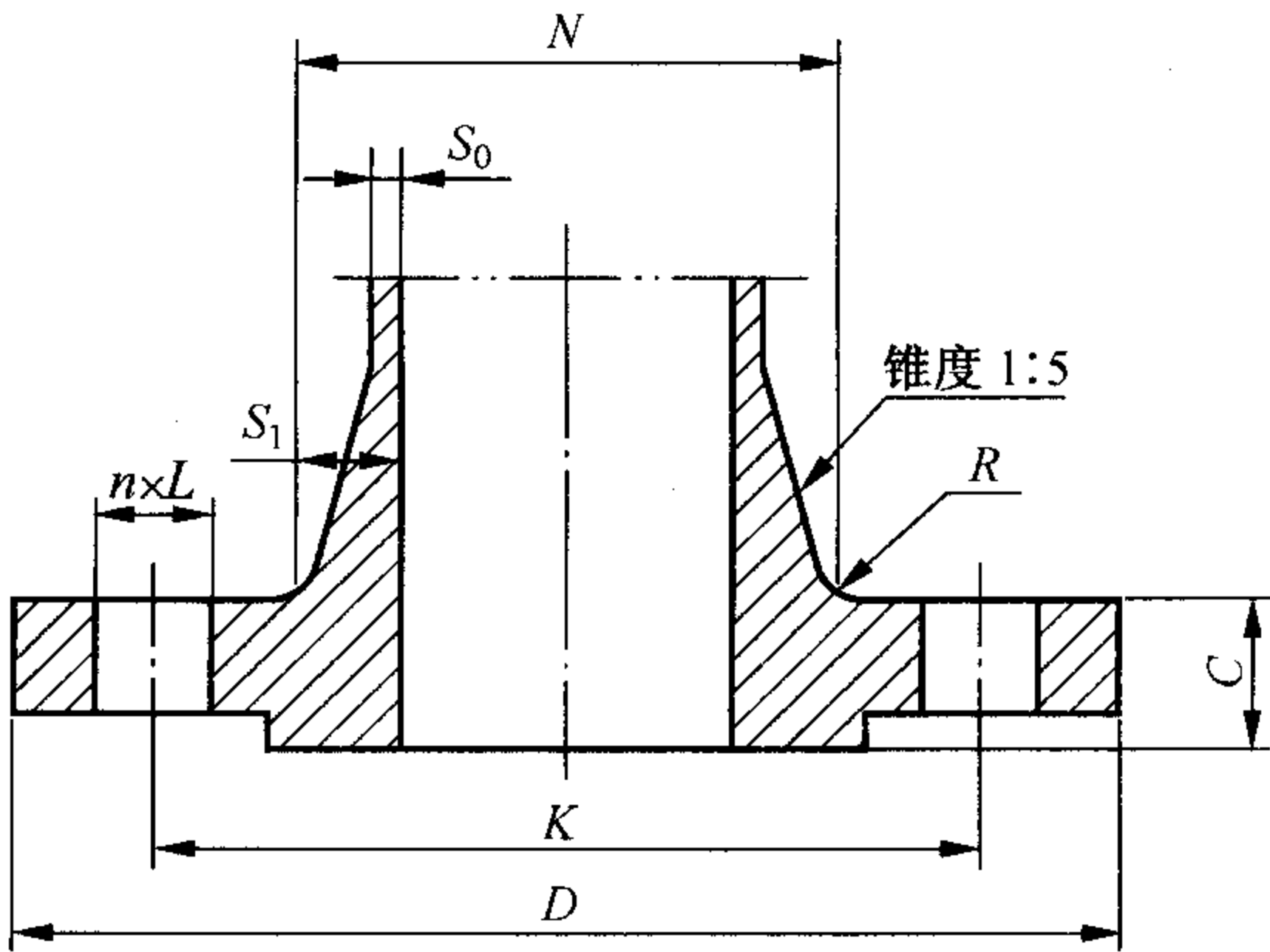
图 8.2.4 整体钢制管法兰
