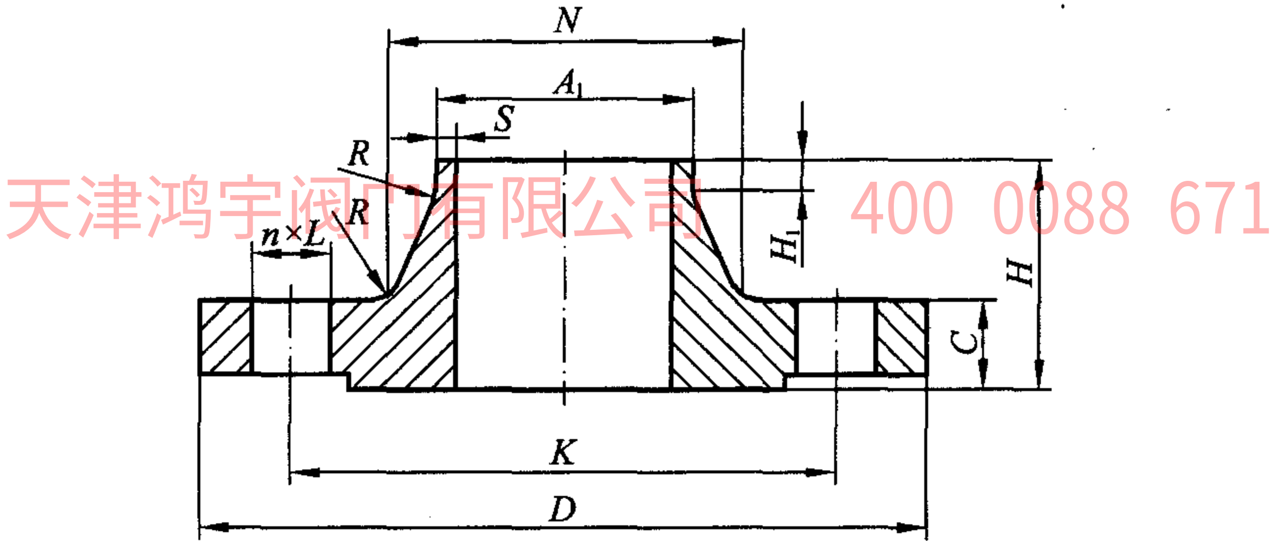
图 8.2.3 带颈对焊钢制管法兰 表 8.2.3-1 PN10 带颈对焊钢制管法兰 (mm)
