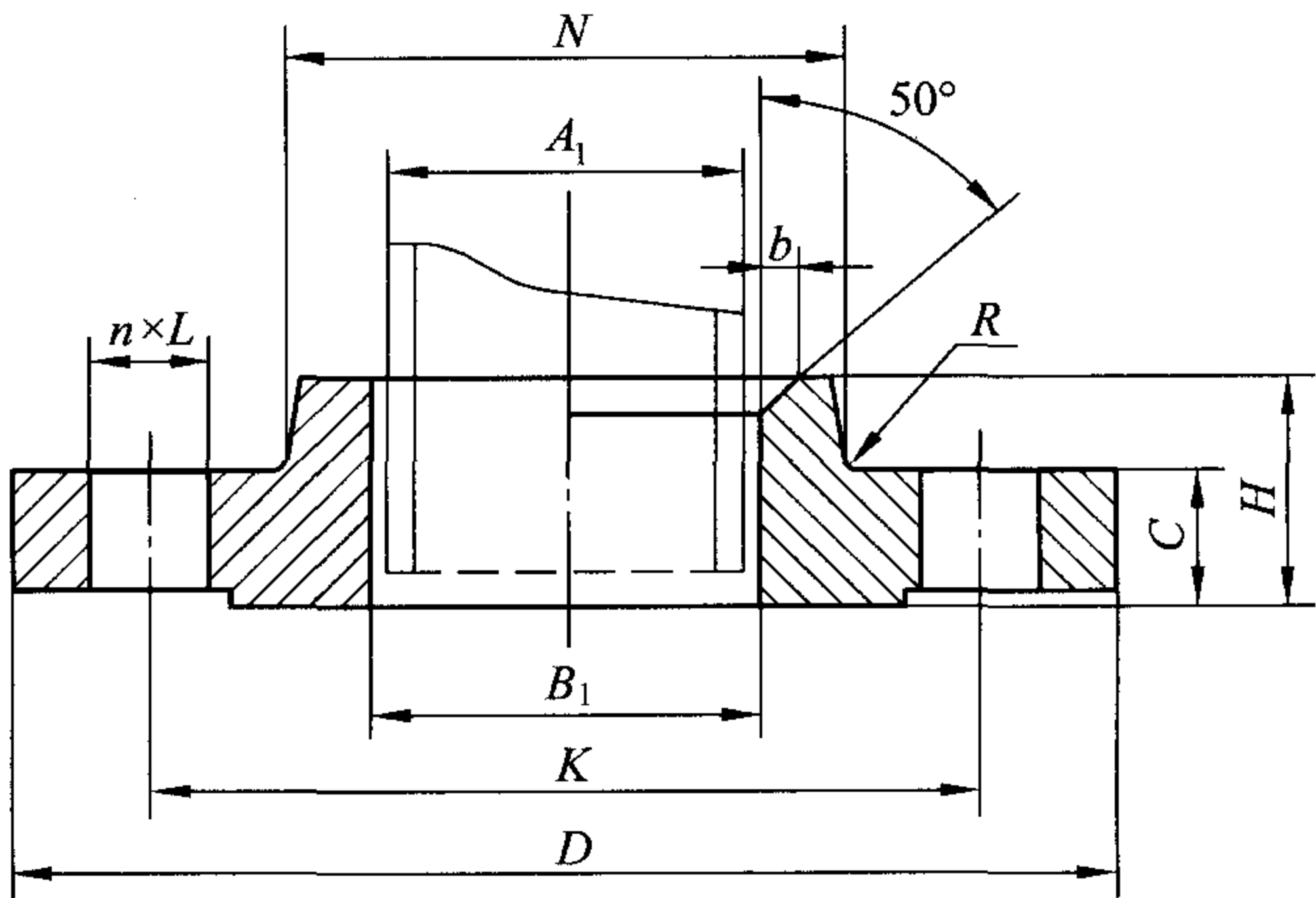
图 8.2.2 带颈平焊钢制管法兰
