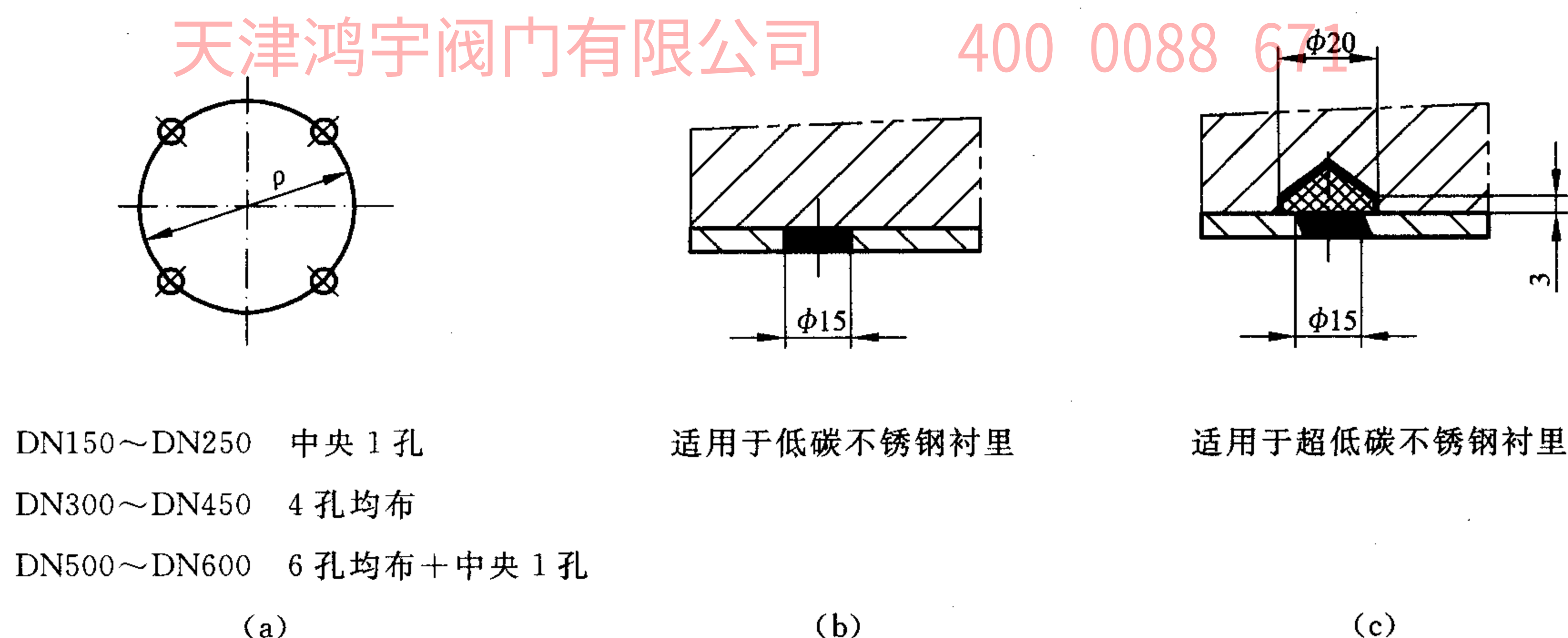
图 4.0.4 衬里法兰盖的塞焊
